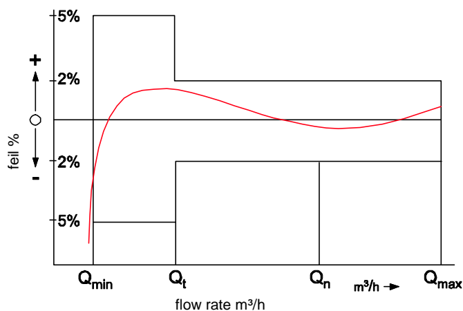
Typisk målenøyaktighetskurve
